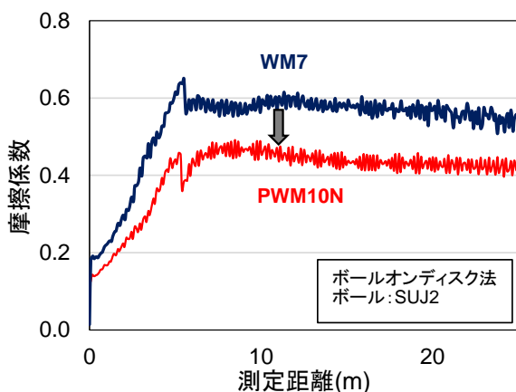
PWM10NはWM7と比較して低摩擦化が図られています
