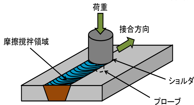
FSW(摩擦攪拌接合)の模式図
