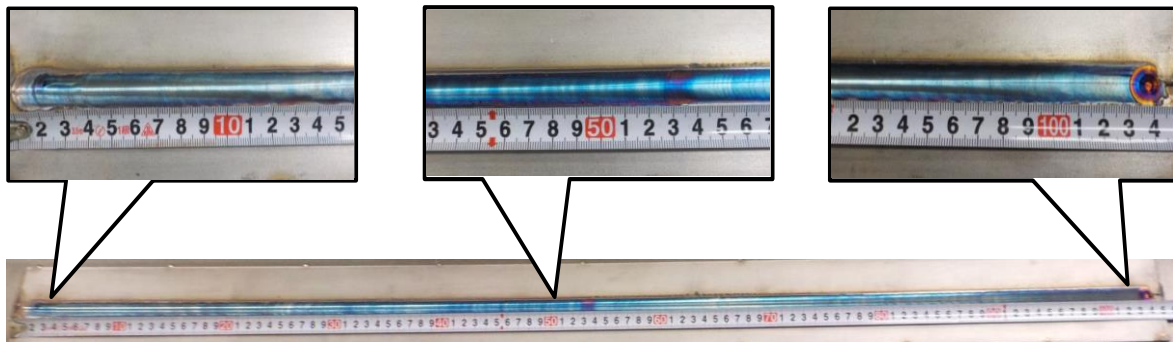
SUS304のFSW(摩擦攪拌接合)実施事例
