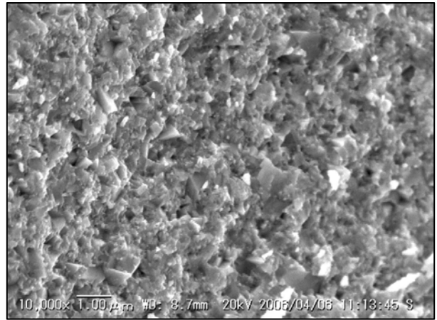
Nano UK 破面 (SEM 組織)
