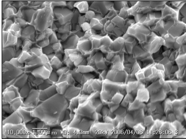
通常材 RD 破面 (SEM 組織)
