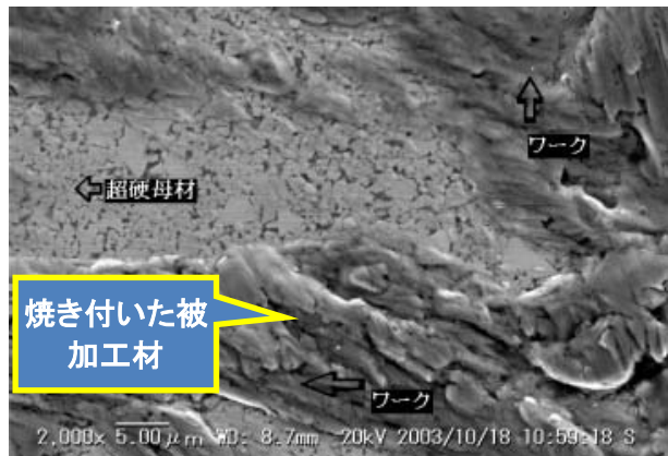
通常超硬型表面への焼き付き事例
