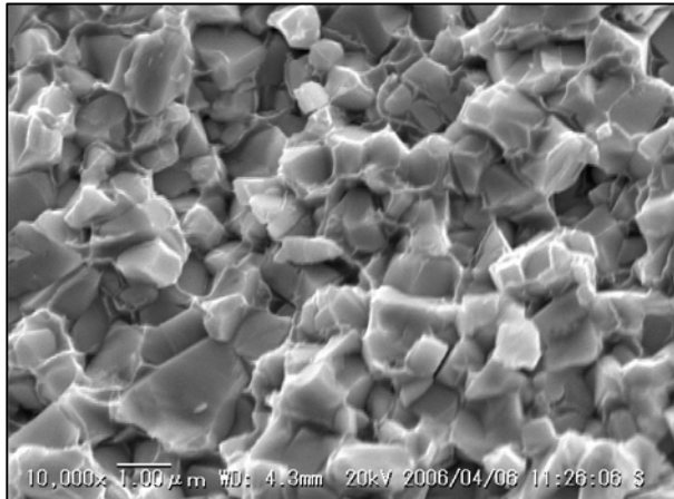
一般RD材料组织 ( SEM组织 )
