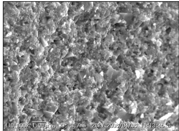
NANO UK 材料组织 ( SEM 组织 )
